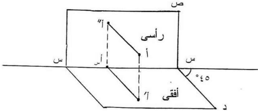
شكل (١-٢) : المسقطين الرأسى والأفقي
