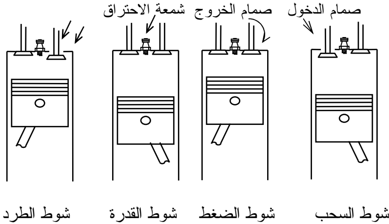
شكل (١٢-٢) : أشواط الدورة الرباعية
