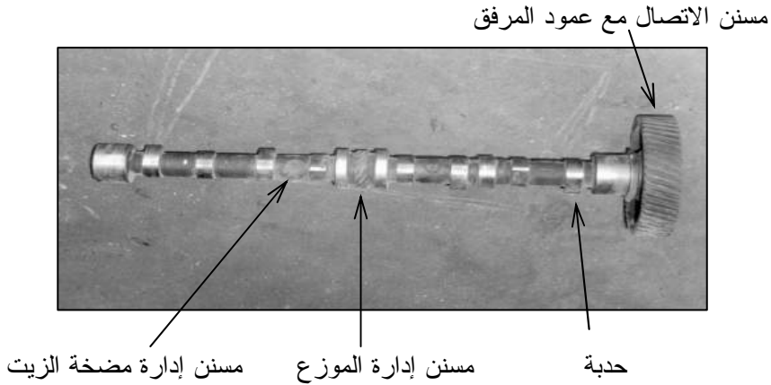
شكل (٢-٢٠) : عمود الحدبات
