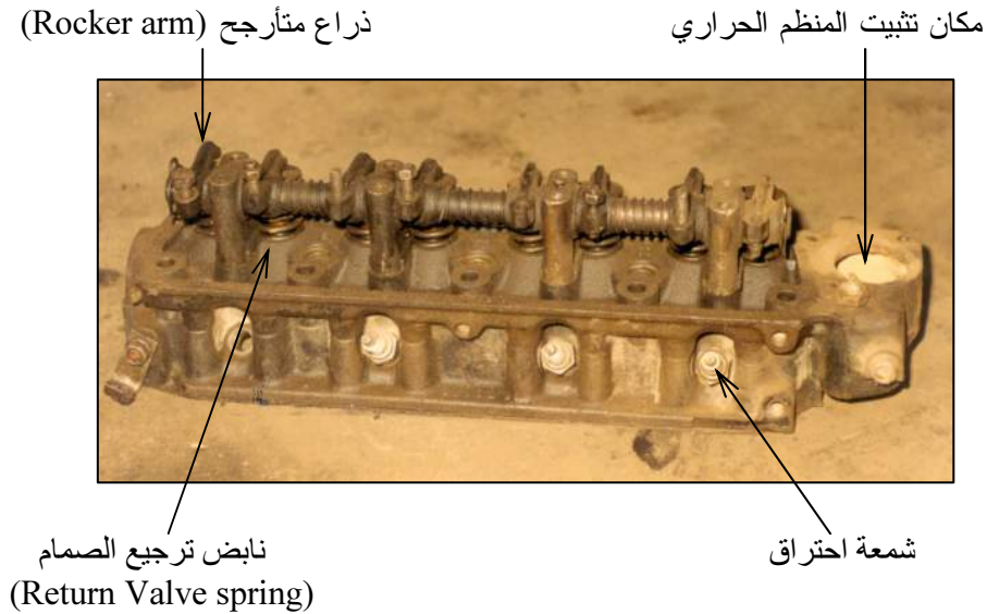
شكل (٢-١٥) : رأس الأسطوانات
