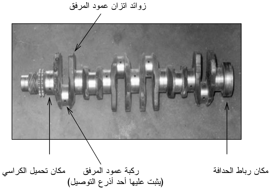
شكل (٢-١٩) : أجزاء عمود المرفق
