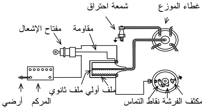
شكل (٢-١١) : رسم تخطيطي يبين مجموعة الإشعال
