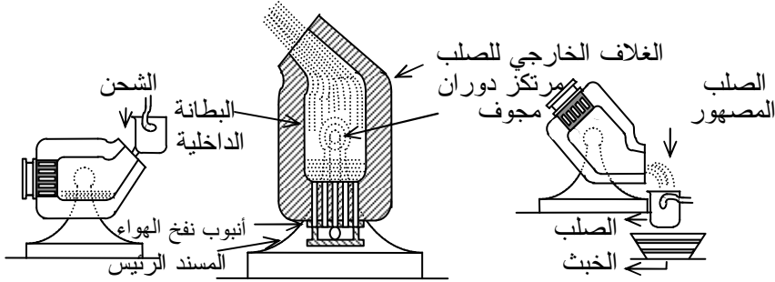
شكل (٢-٤) : محول بسمر
